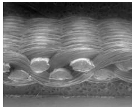
Flowrox W-TA220L toile filtrante image au microscope électronique
